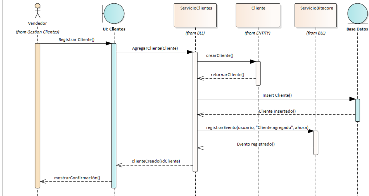
sd DiagramaSecuenciaGestionClientes
