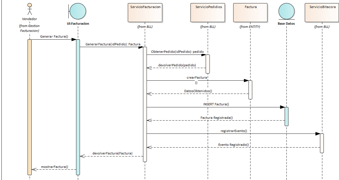
sd DiagramaSecuenciaGestionFacturacion
